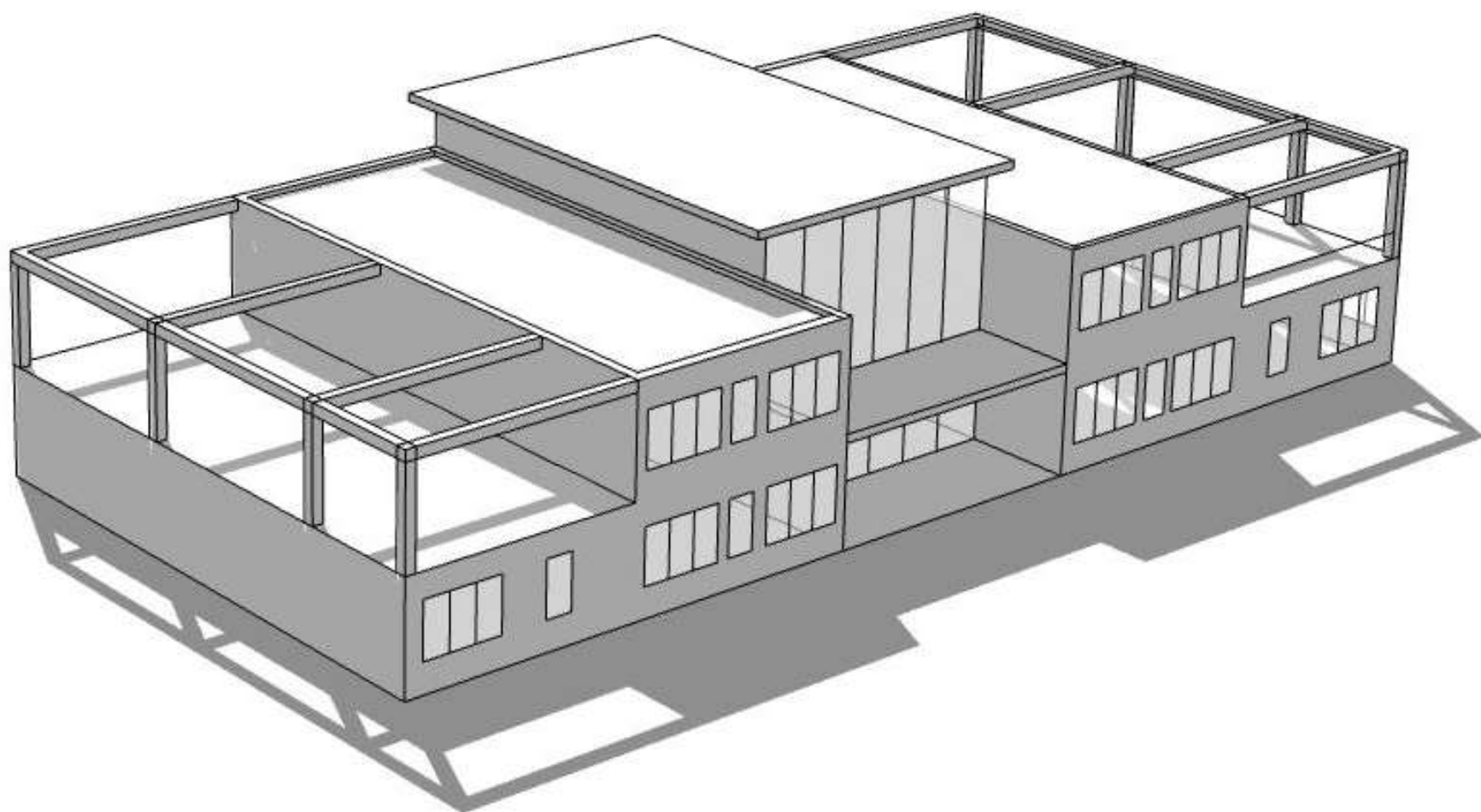
VISTA ASSONOMETRICA 2
